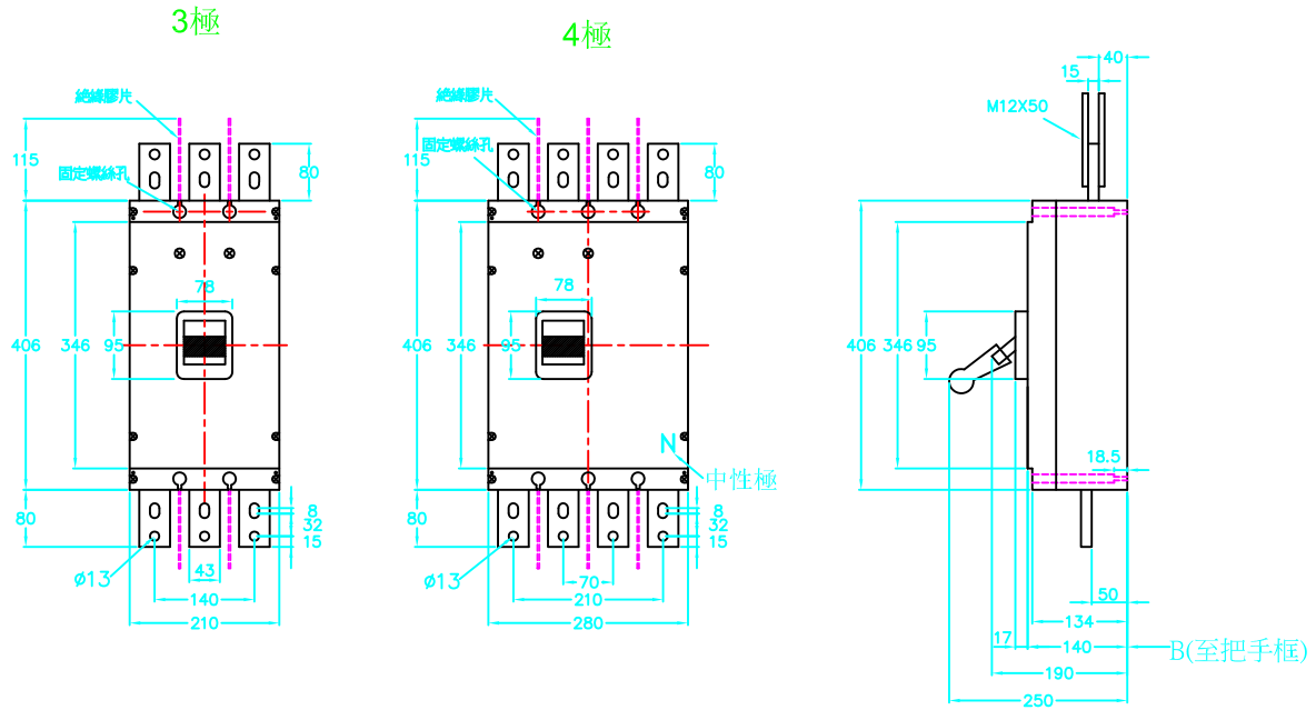
B:底板鑽孔攻牙及面板挖孔尺寸圖 (至把手框)
