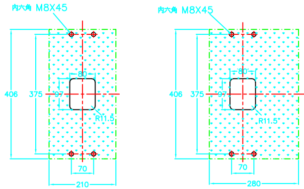
C:背接外型尺寸及底板鑽孔攻牙尺寸圖
