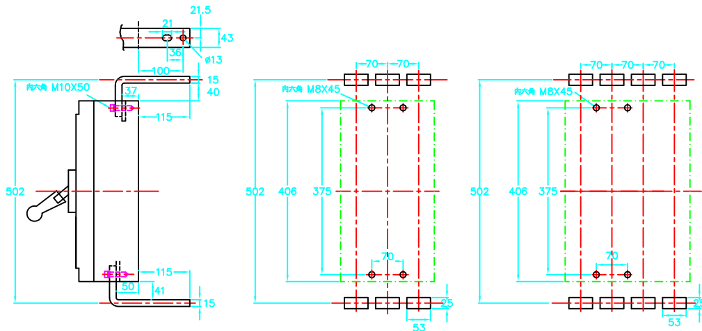
C:背接外型尺寸及底板鑽孔攻牙尺寸圖
