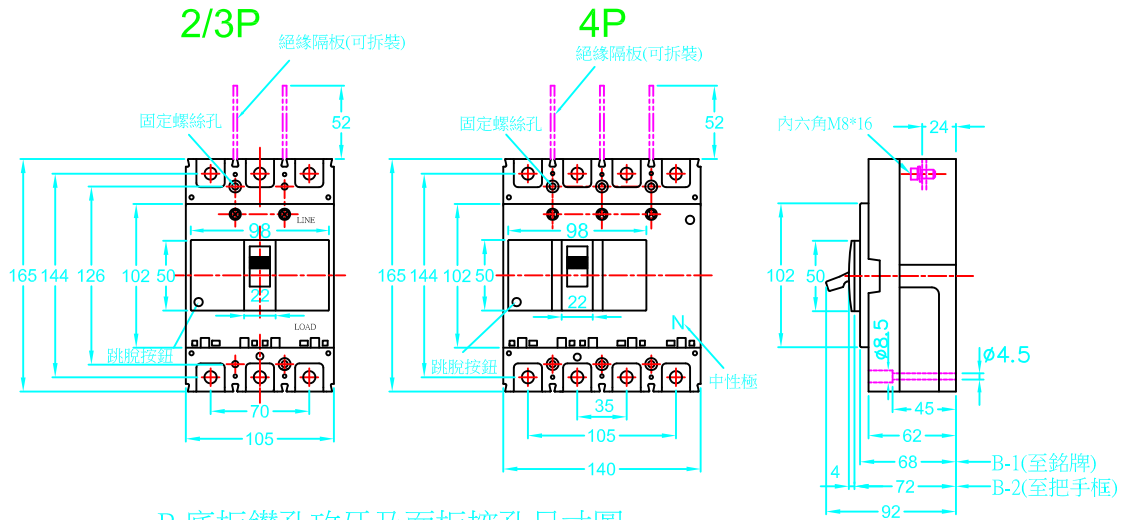
B:底板鑽孔攻牙及面板挖孔尺寸圖
