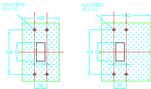
C:背接外型尺寸及底板鑽孔攻牙尺寸圖
