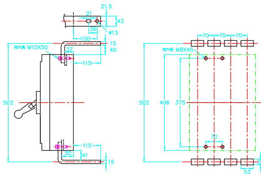
C:背接外型尺寸及底板鑽孔攻牙尺寸圖
