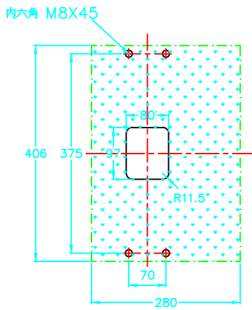
C:背接外型尺寸及底板鑽孔攻牙尺寸圖
