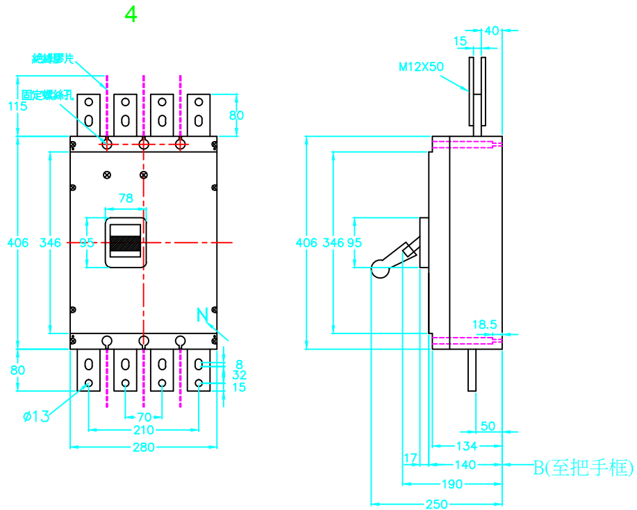
B:底板鑽孔攻牙及面板挖孔尺寸圖 (至把手框)
