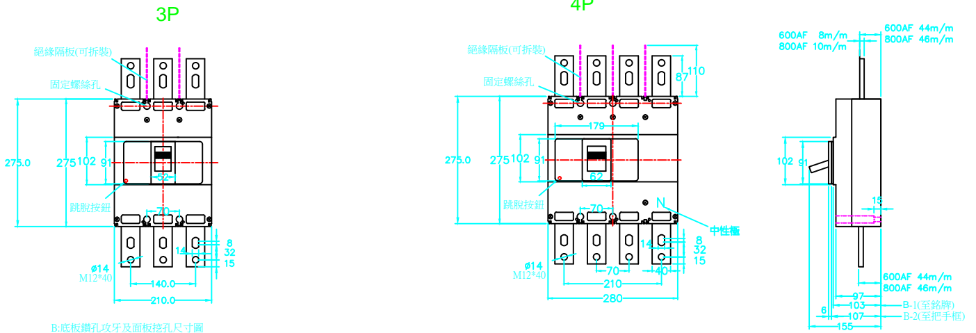
B:底板鑽孔攻牙及面板挖孔尺寸圖 B-1(至銘牌)
