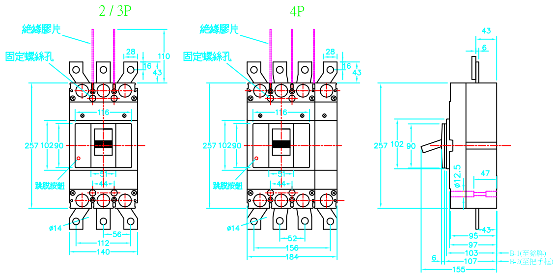
B:底板鑽孔攻牙及面板挖孔尺寸圖
