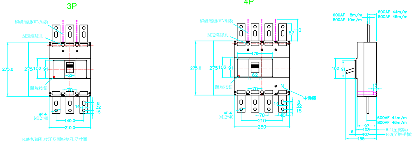
B:底板鑽孔攻牙及面板挖孔尺寸圖
