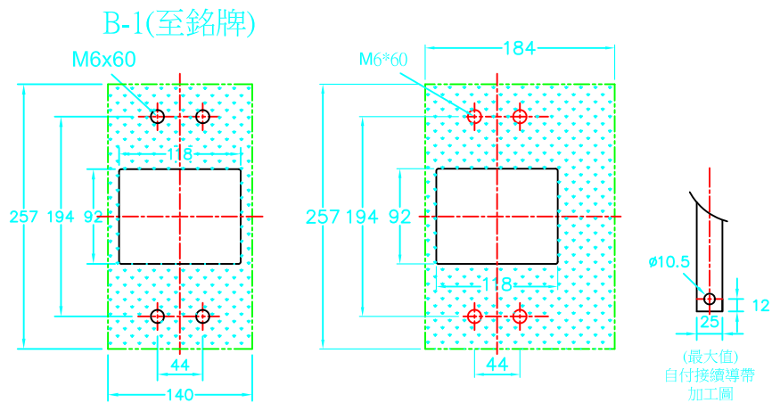
B:底板鑽孔攻牙及面板挖孔尺寸圖
