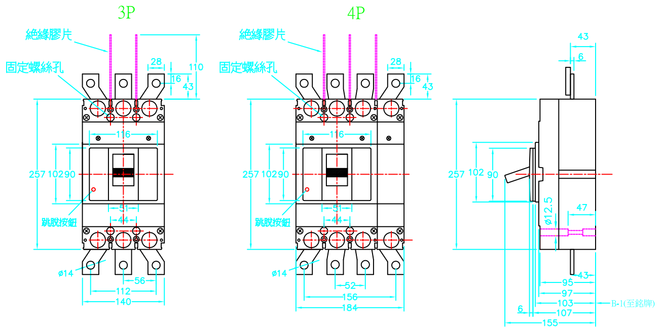
A:外型尺寸圖
