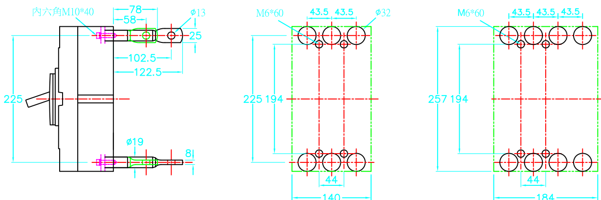
C:背接外型尺寸及底板鑽孔攻牙尺寸圖
