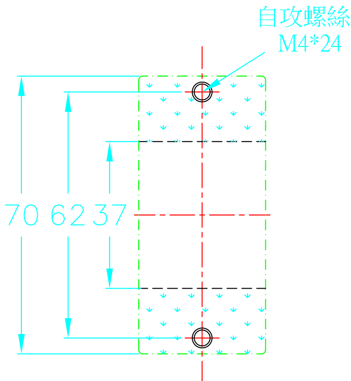
B:底板鑽孔攻牙及面板挖孔尺寸圖
